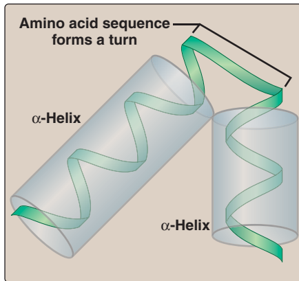
Figure 32.5 Helix-turn-helix motif.
